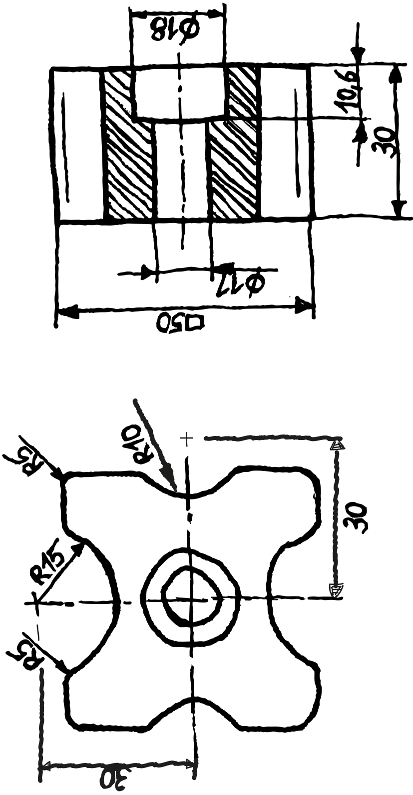
Gelenkstück
