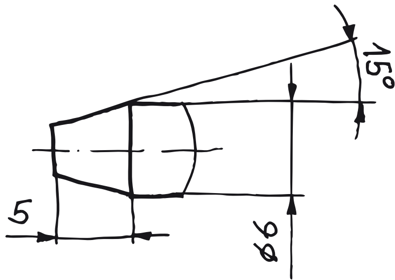
Anschlagnadel
